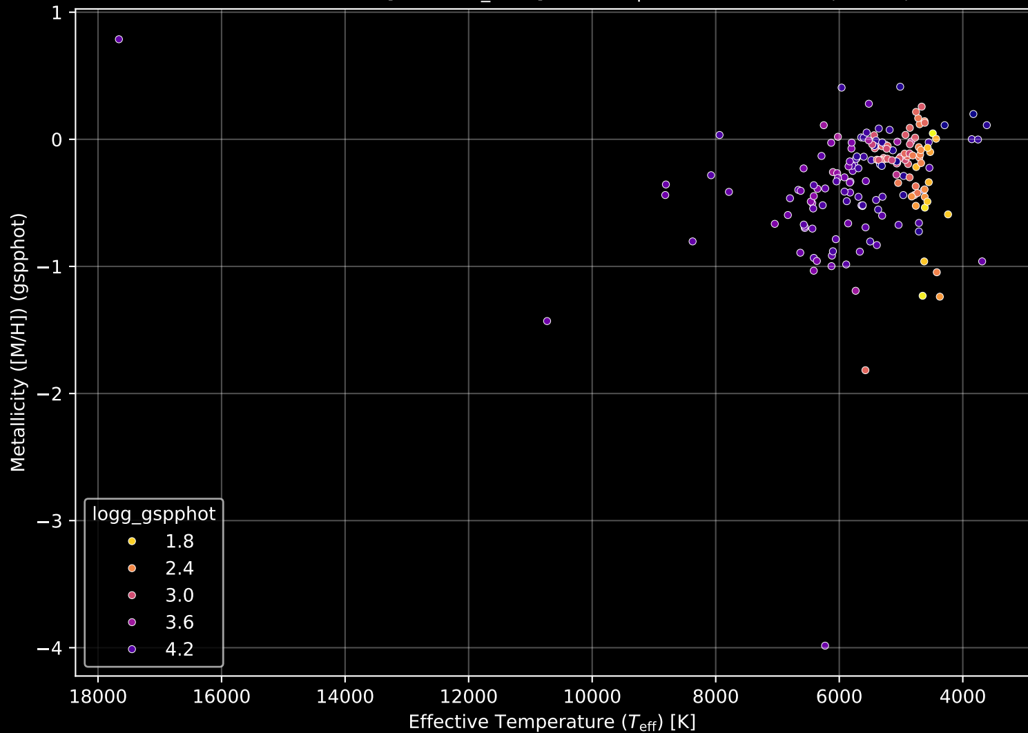
APOGEE DR17 Field: [274-18-O_TESS] Stellar Population Parameters (n= 176)
